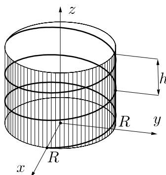
Rys. 1.12. Linia śrubowa
