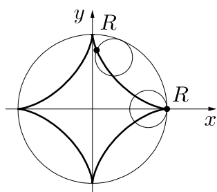
Rys. 1.10. Asteroidea
