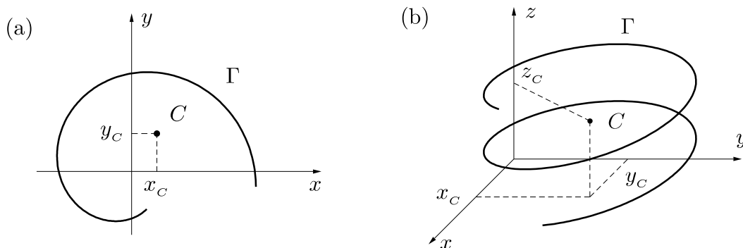
Rys. 1.17. Współrzędne środka masy łuku: (a) na płaszczyźnie; (b) w przestrzeni
